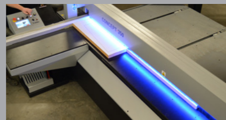
Statusanzeige Blau: Maschine sägt
