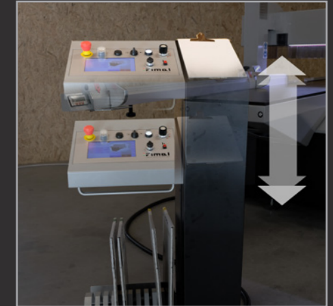
Höhenverstellbares Bedienpult, kann unter Tischhöhe oder über den Teleskopanschlag gefahren werden
